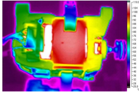
UMAC Motor
